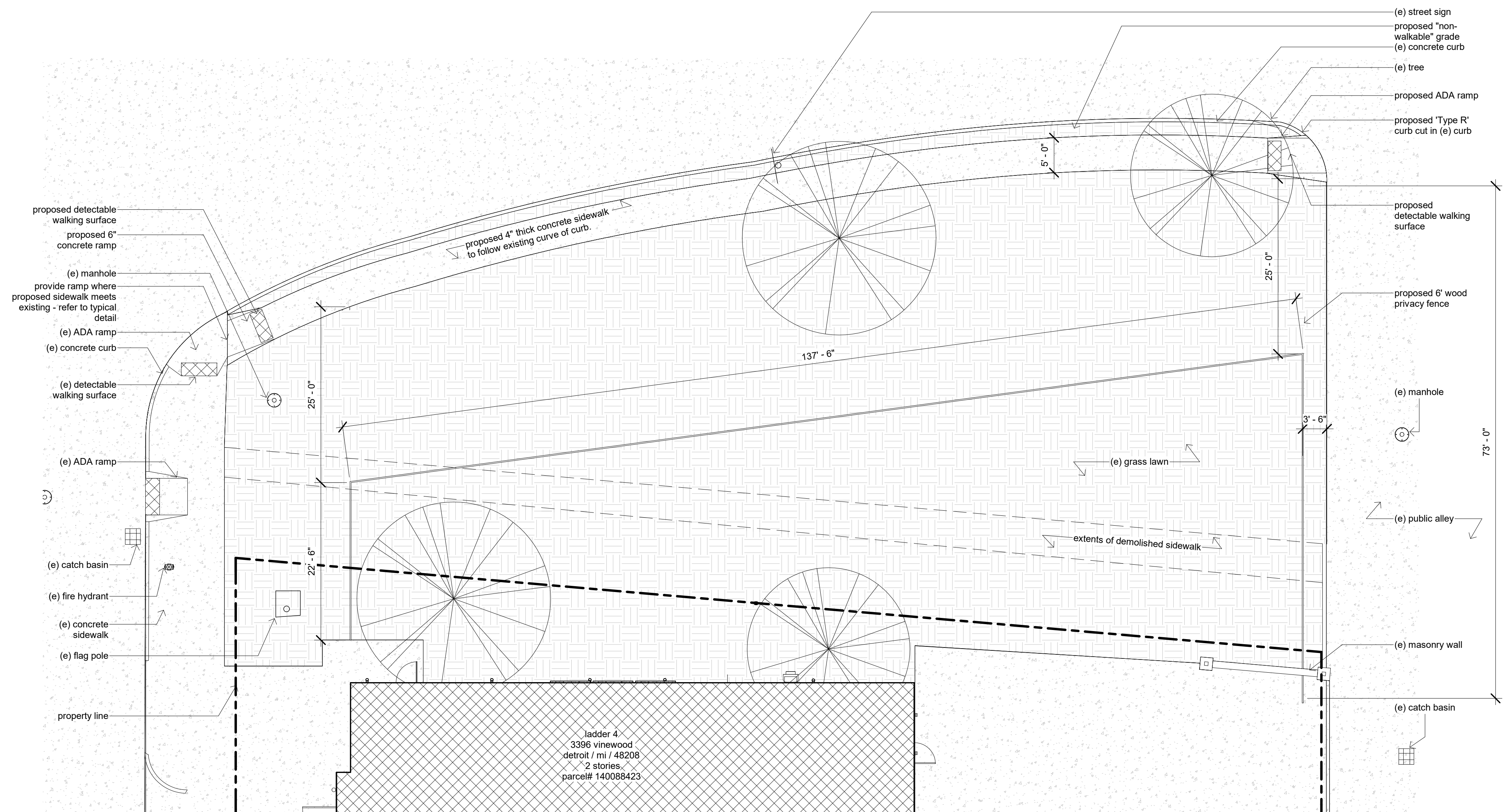
legend / site plan 11
