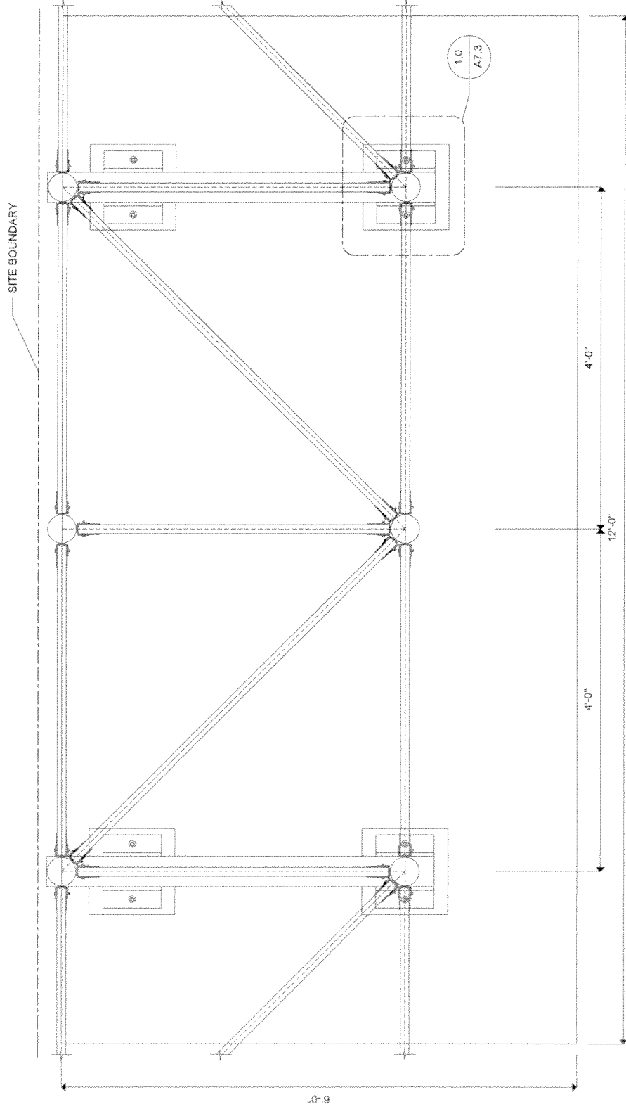
1.0 F1 FOUNDATION DETAIL
