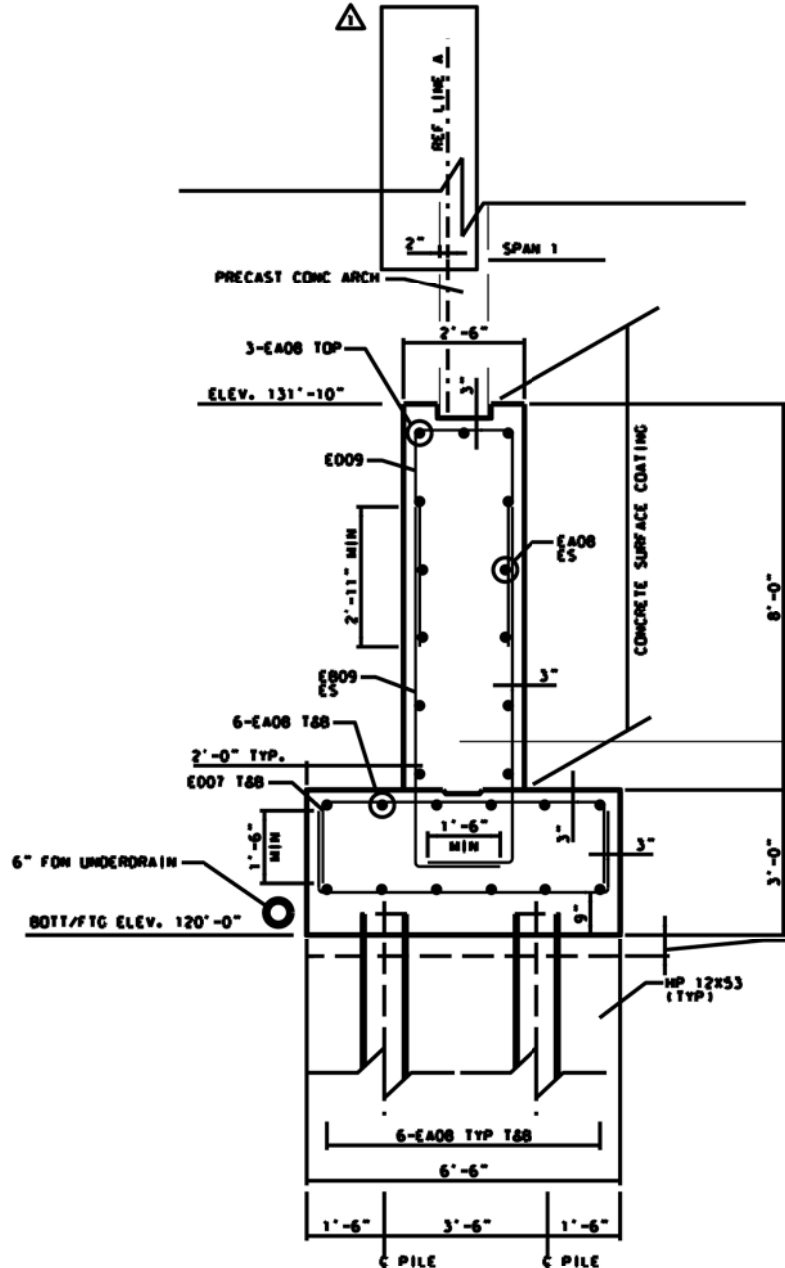
SECTION E-E SCALE: 1/2" = 1'
