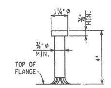
STUD DETAILS
