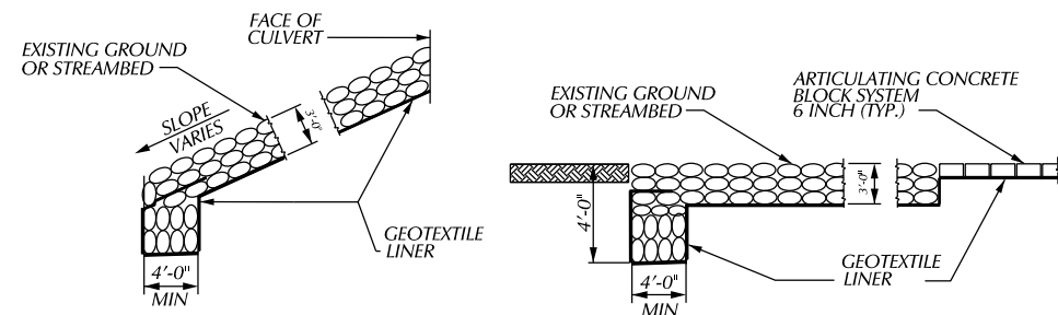
TOE HEADER
