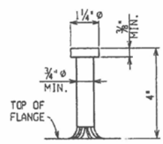
STUD DETAILS
