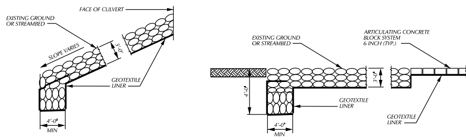
TOE HEADER
