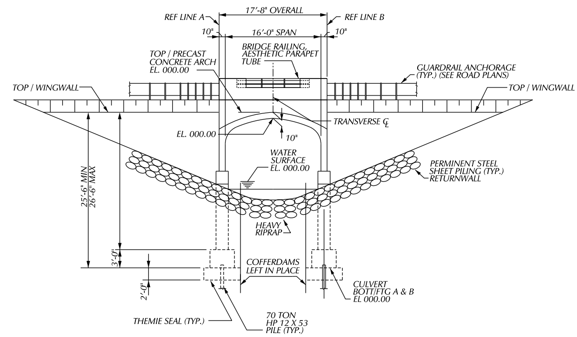
ELEVATION
